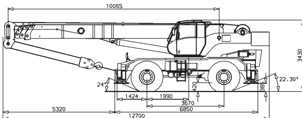
Dimensioni (mm)
